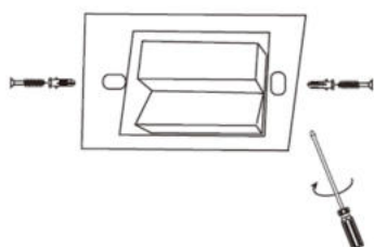
4. Fije el luminario.
