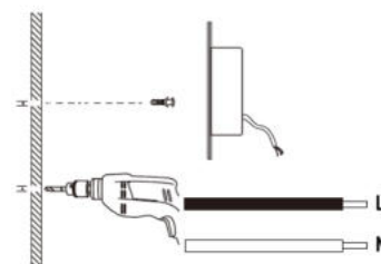
3. Haga perforaciones en la superficie para fijar el luminario.
