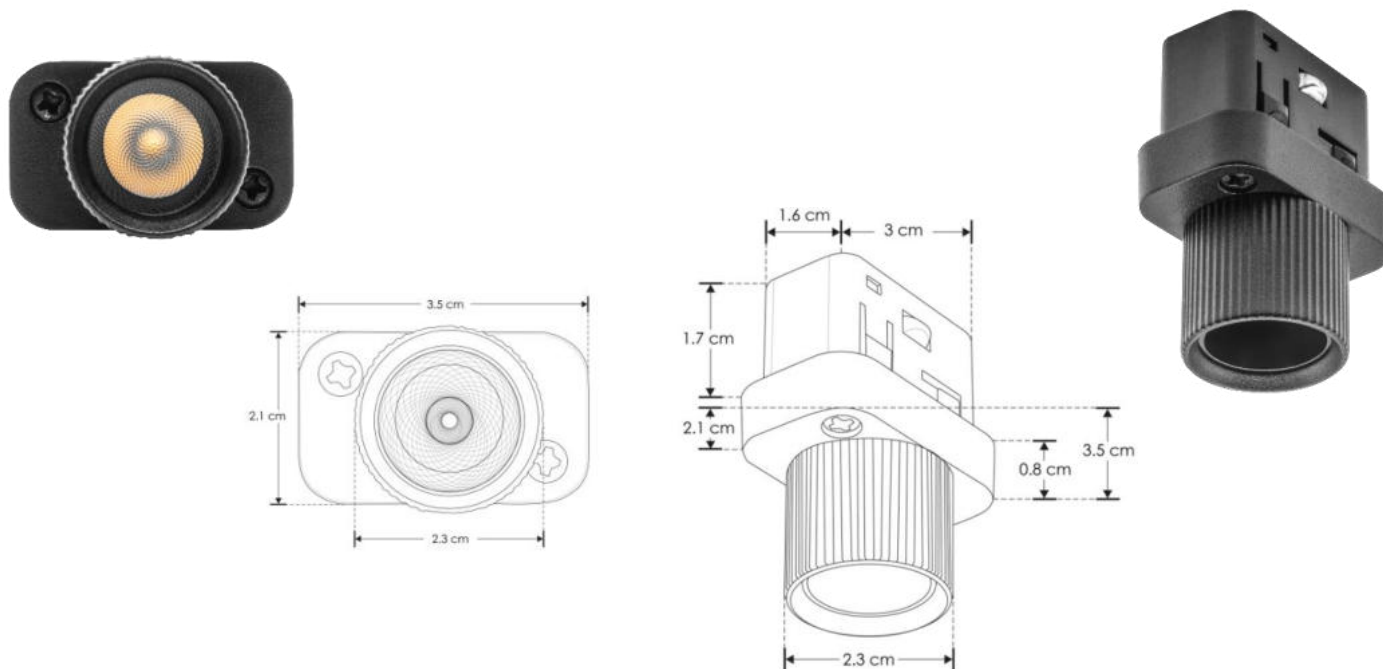
Luminario de LED con UGR 19
