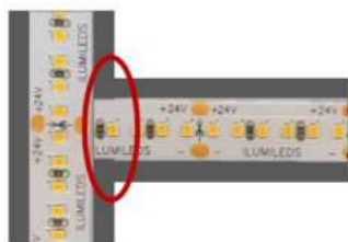
Intersección en perfil con ceja lateral
