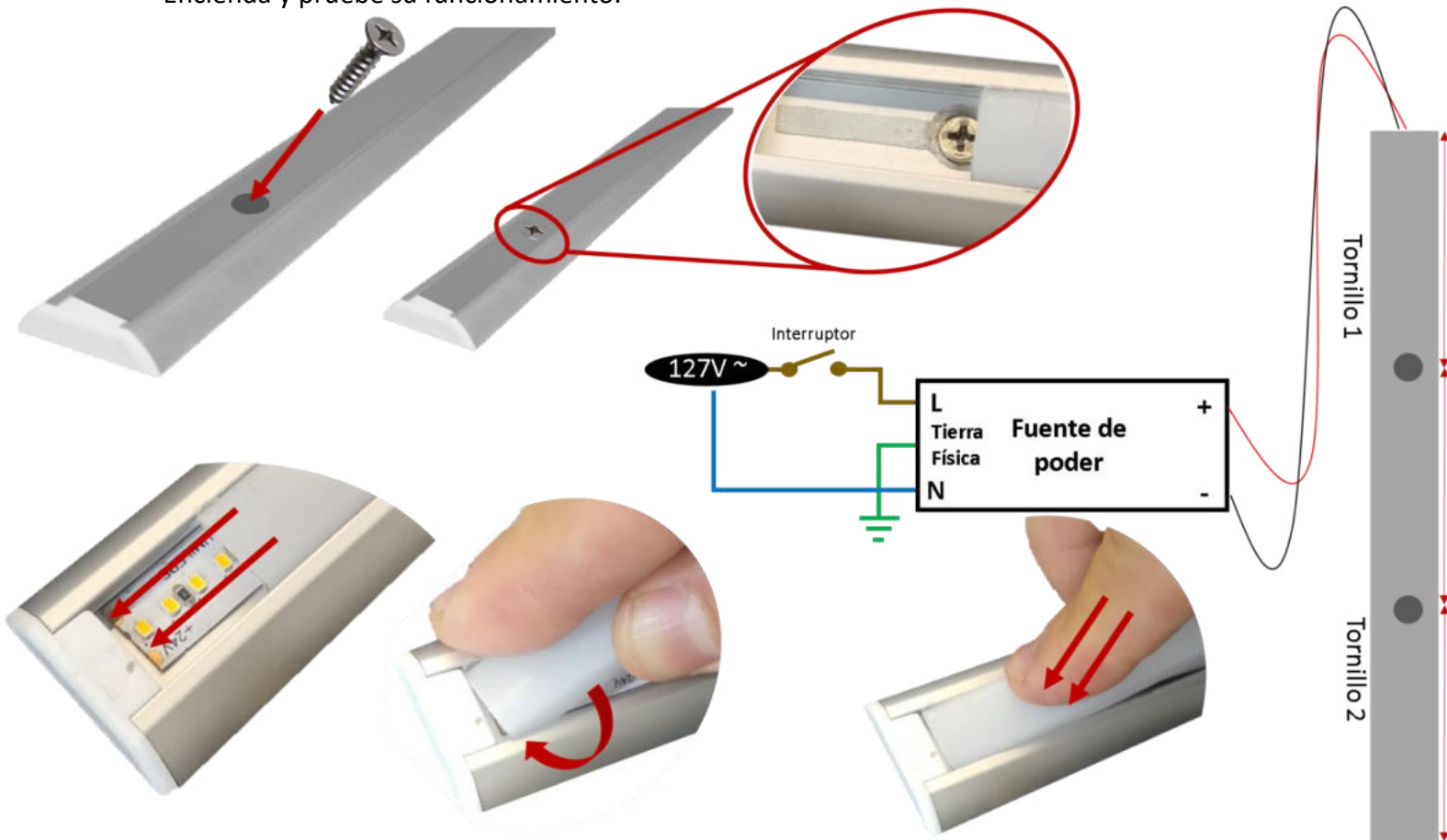
Fijación directa (avellanado)
