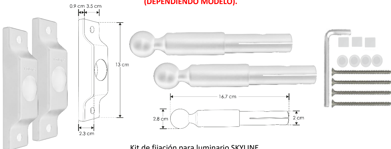
Kit de fijación para luminario SKYLINE
