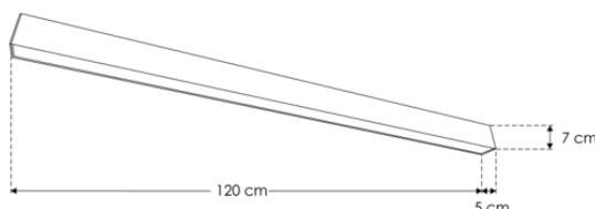
ILUINTB120CMWWB, ILUINTB120CMNWB
